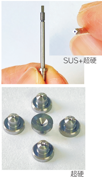
吸着ノズル
