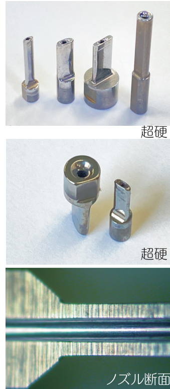
巻線ノズル
